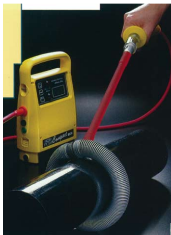
管外測頭
